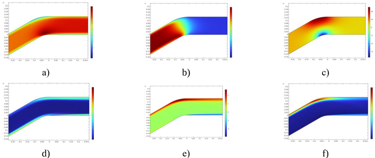
Fig. 9 Isolines a) longitudinal velocity -U , b) transverse velocity -V , c) pressure -p , d) \overline{u'u'} , e) \overline{v'v'} , f) \overline{u'u'} .
